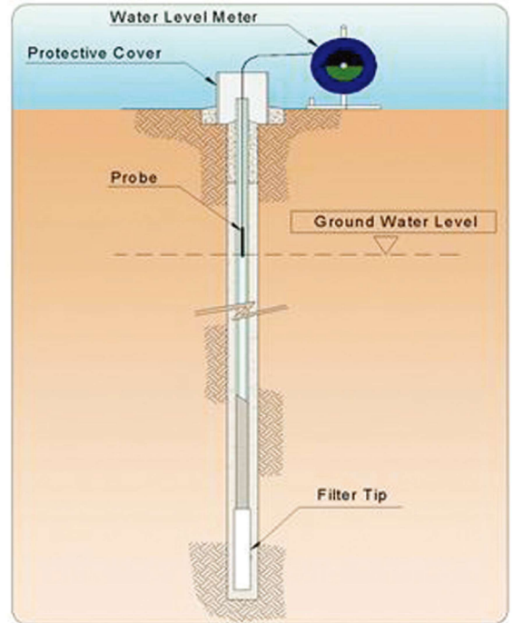
[모델 4650 설치도]
